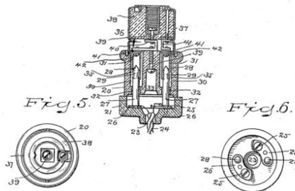
Tekening van eerste elektrische stopcontact (VS-patent: 774,250)
